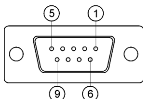
Connettore D-Sub femmina a 9 poli
