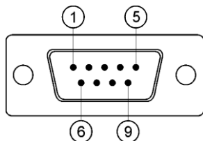
Connettore D-Sub a 9 poli
