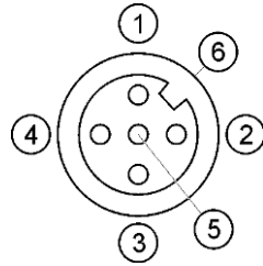
M12-втулка: Ethernet
