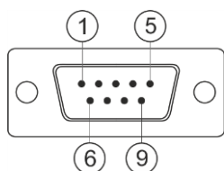
9-полюсный Sub-D-штекер
