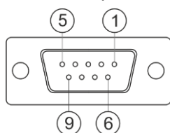
9-Контактная Sub-D-розетка
