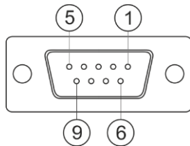
Fișă D-Sub cu 9 poli
