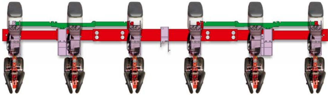
A vetőelemek elrendezése a TELESZKÓPOS PROSEM K (250/6) vetőgép változaton
