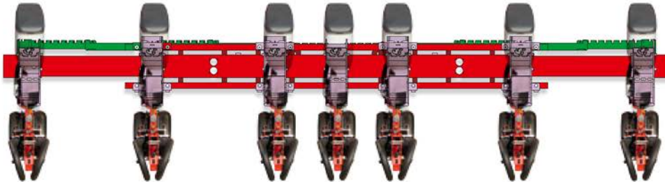
A vetőelemek elrendezése a PROSEM K VARIANT (300/7S) vetőgép változaton
