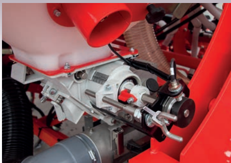
Distributor volumetric, usor de reglat pentru toate tipurile de seminte
